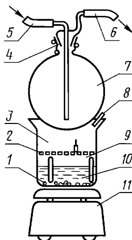
Установка для ускоренного старения в водяном паре
