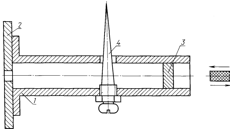
1 - волновод (10Ч23); 2 - диафрагма; 3 - поршень настройки; 4 - антенна
