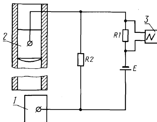
1 - наковальня (основание); 2 - боек (стол); 3 - осциллограф
