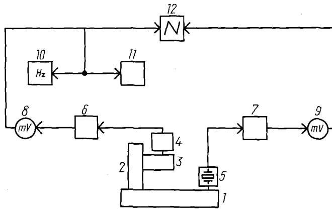
1 - стол вибростенда; 2 - приспособление для испытаний; 3 - испытуемое изделие; 4 - электретный вибропреобразователь; 5 - пьезоэлектрический вибропреобразователь; 6, 7 - катодные повторители; 8, 9 - милливольтметры; 10 - частотомер; 11 - самописец; 12 - осциллограф
