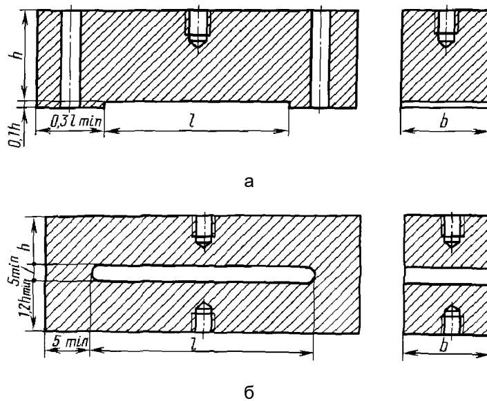
а - точки крепления балки расположены по бокам; б - точка крепления балки расположена в центре
